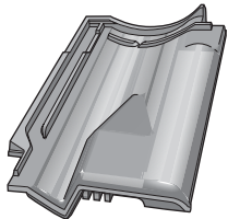
Ventilationssten med gitter, helt i tegl Nr. 741 Udluftning, ca. 15 cm 2
