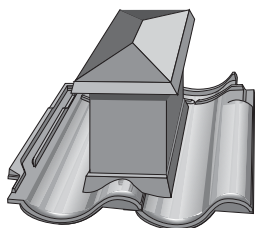
Udluftningshætte med isorør Tagvinkler 20 - 45° Indvendig, ca. 150x150 mm Udluftning, ca. 225 cm 2
