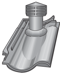
Lodret tudsten, helt i tegl Nr. 750 Til mekanisk udluftning Justerbar til tagvinkler Rørdiameter, ca. 20 - 45° 100 mm
