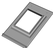
Folieflange Til gennemføring ved undertag Plade til 150x150 mm rør 260x470 mm Åbning 170x230 mm
